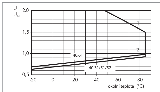
R 40 - pracovní rozsah DC cívek se zvýšenou citlivostí u typu 40.31/51/52/61/62
